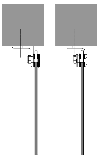
ŘEZ A
