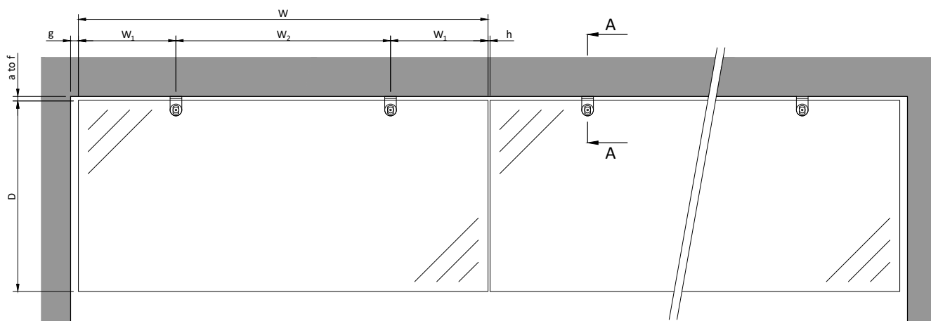
POHLED
